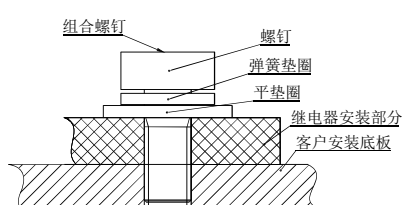
继电器安装
