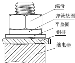
外螺纹
