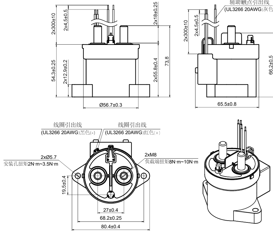
外形图
