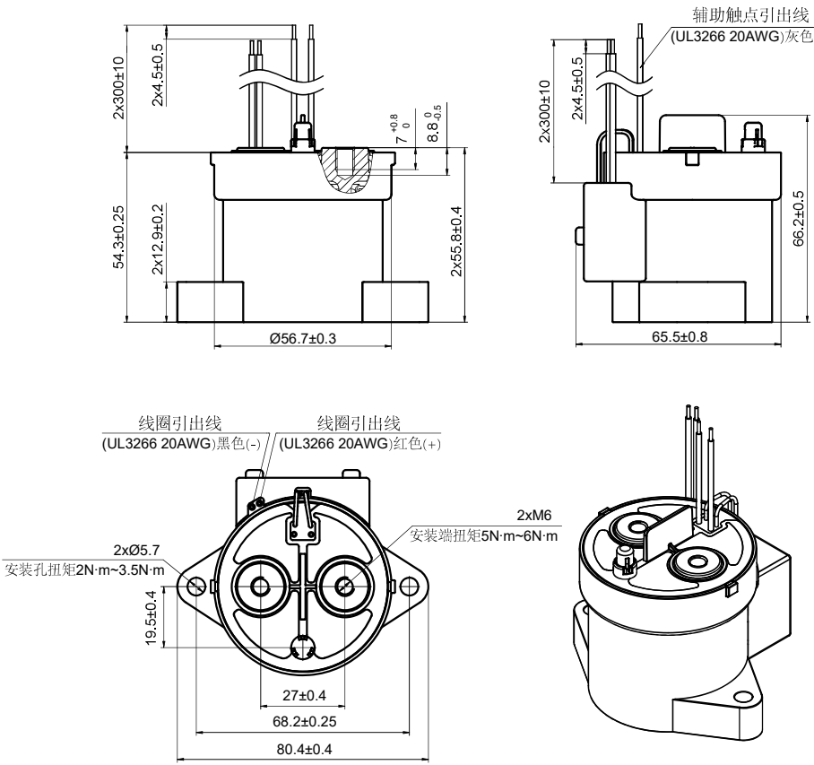
HFZ21-150-B内螺纹
