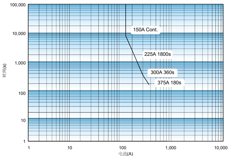
载流能力—通电时间(150A)
