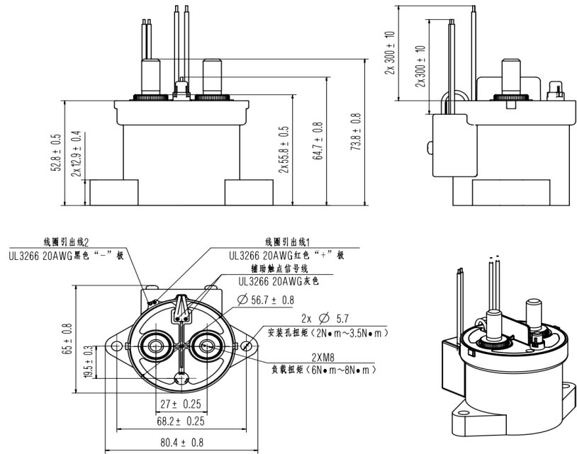
HFZ16-200 外螺纹
