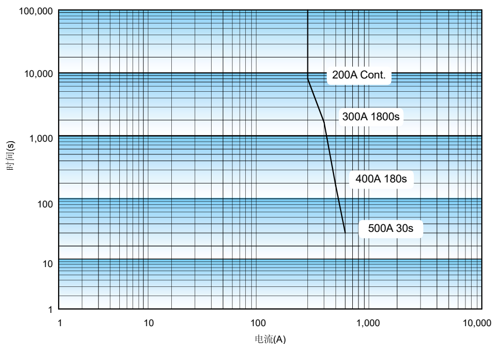
载流能力—通电时间(200A)
