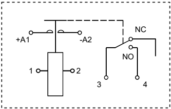
接线图
