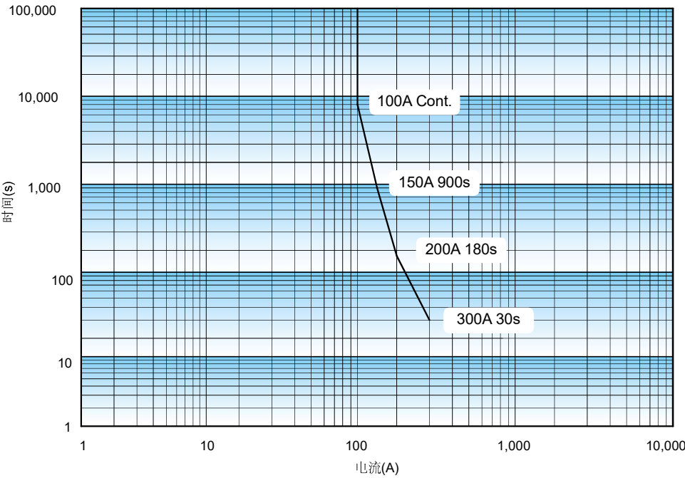
载流能力—通电时间(100A)
